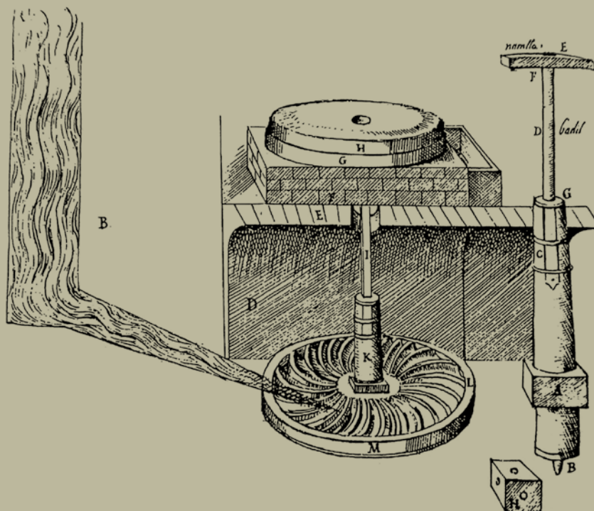
Reproducció d'un molí fariner del segle XVI, de Los veintiún libros de los ingenios y máquinas . Fons de la Biblioteca Nacional d'Espanya, Madrid
